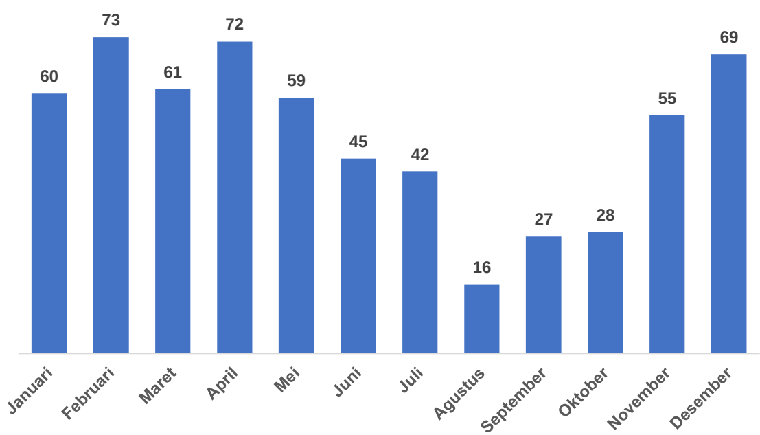
Gambar 2.4 Jumlah Hari Hujan Kabupaten Penajam Paser Utara Menurut Bulan Tahun 2023
