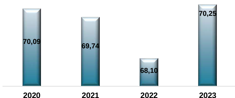
Gambar 2.53 Indeks Kualitas Lingkungan Hidup Tahun 2020 – 2023
