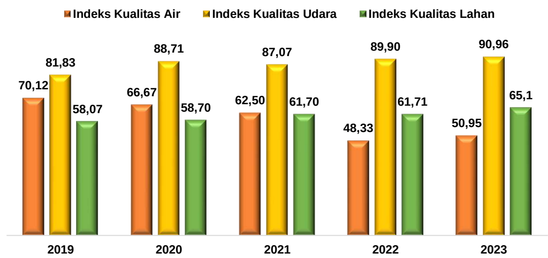
Gambar 2.52 Indeks Kualitas Air, Udara dan Tutupan Lahan Tahun 2019–2023
