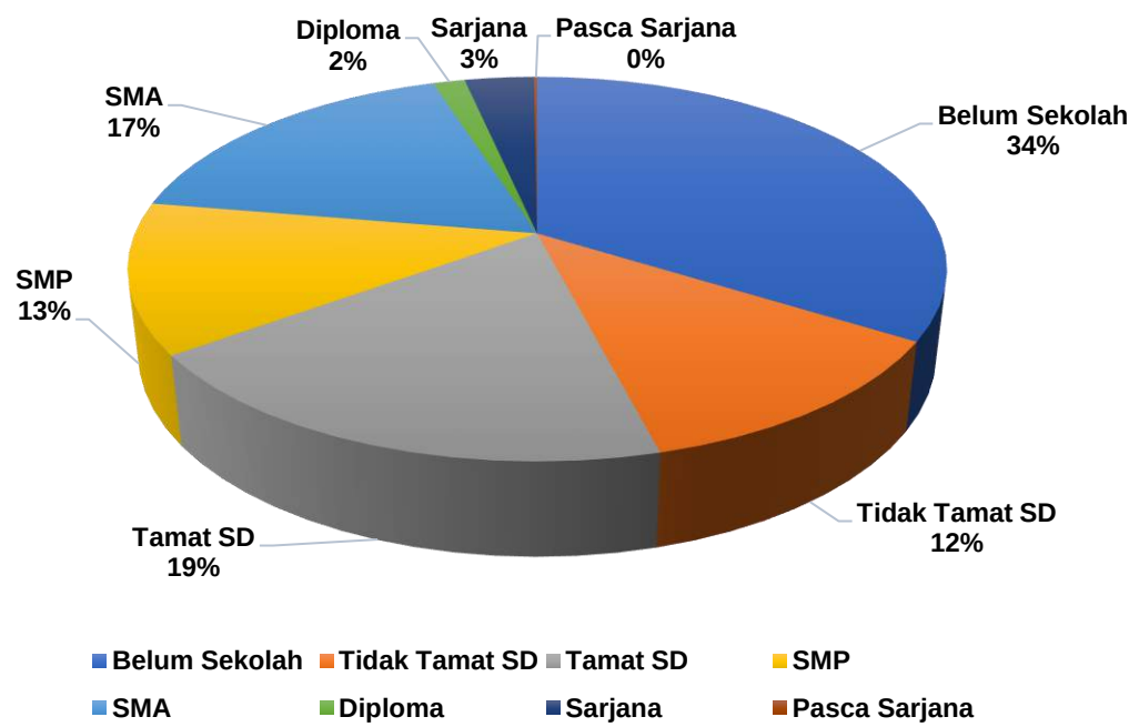
Gambar 2.91 Persentase Tingkat Pendidikan Penduduk Tahun 2023
