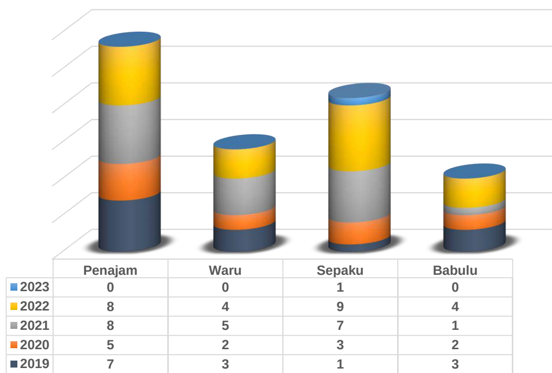
Gambar 2.11 Jumlah Kasus Bencana Banjir Tahun 2019 – 2023
